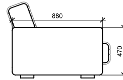
elevação lateral
