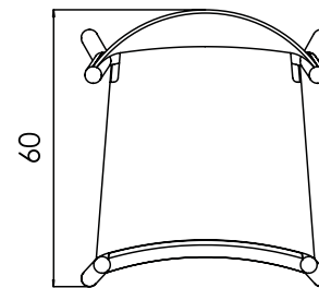
elevação superior
