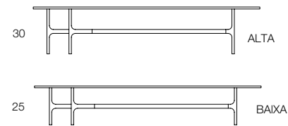
elevação lateral
