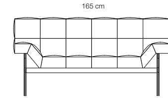
elevação frontal
