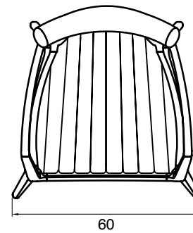
elevação superior
