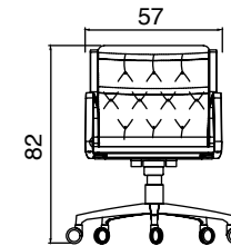
elevação frontal
