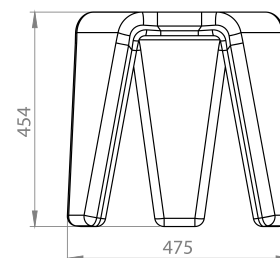
elevação frontal
