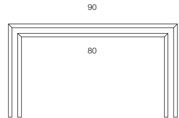
elevação frontal
