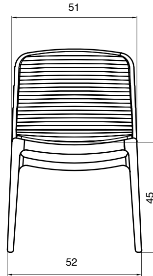
elevação frontal
