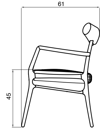
elevação lateral
