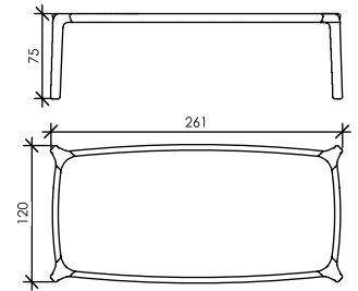
elevação lateral
