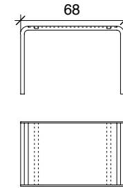
elevação frontal
